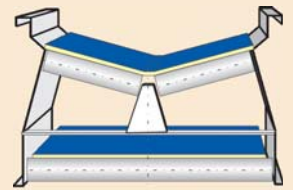
Aufbau RB 500 / RB 650
