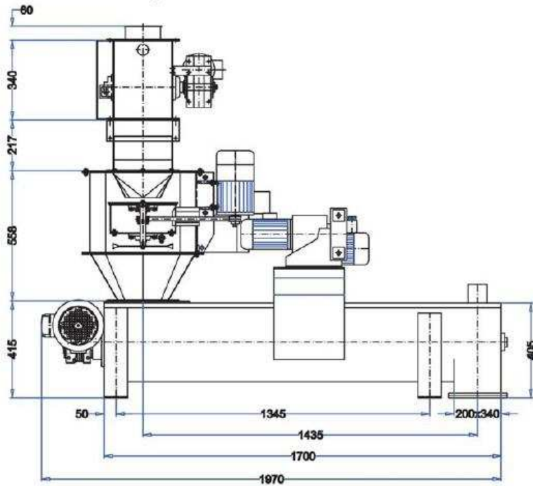
Cellás adagolóval és szelelővel
